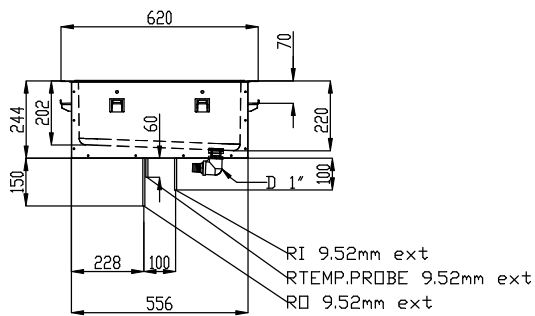
Zij aanzicht
