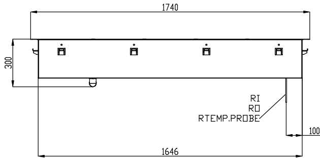
Zij aanzicht
