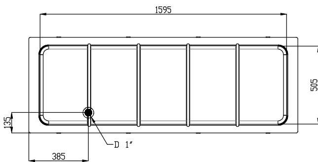
Boven aanzicht
